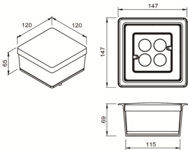
預埋盒 Embedded box
